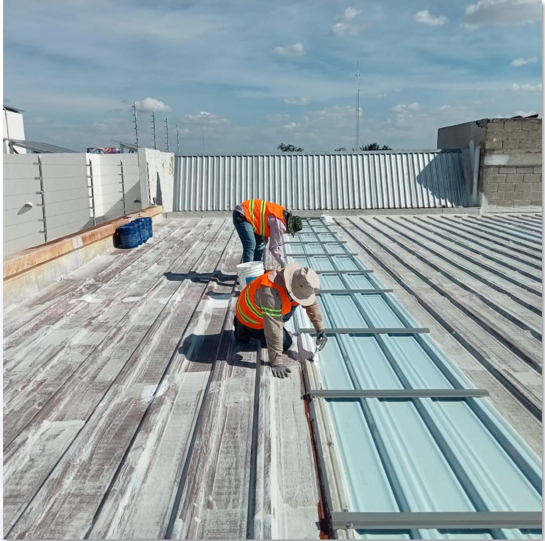
Sellado de los puntos críticos
